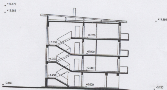
REZ A-A
