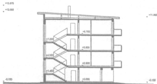
REZ A-A
